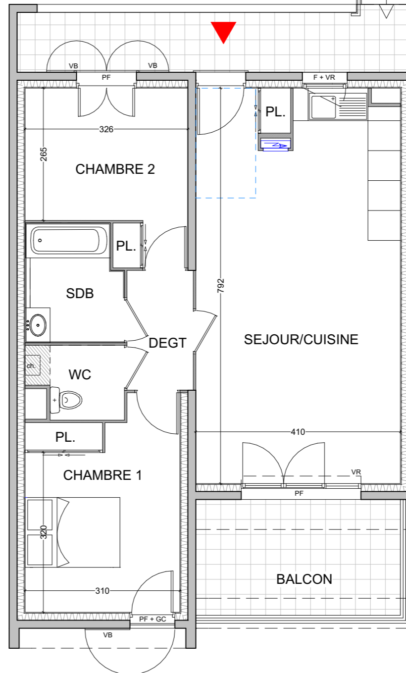
PLAN DE R+1
