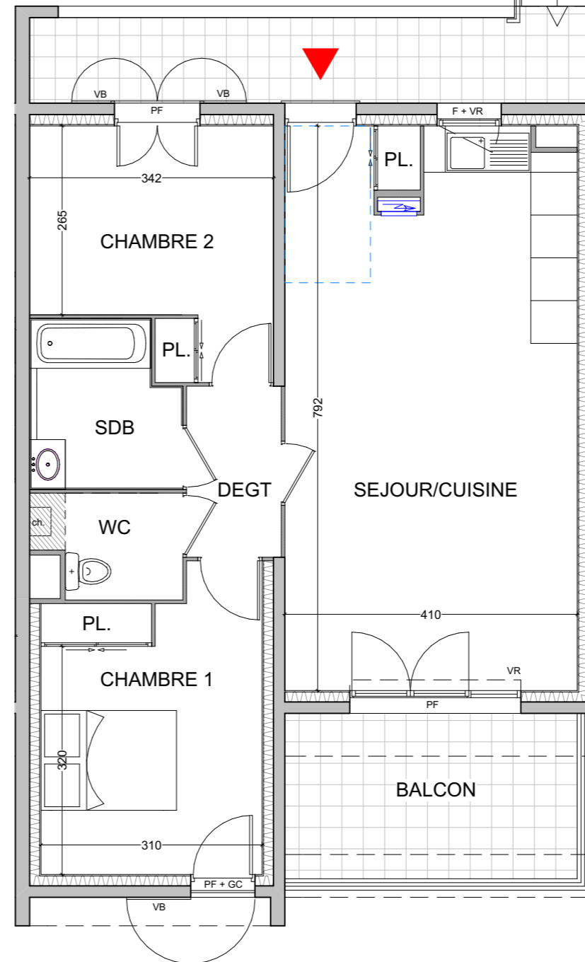
PLAN DE R+1
