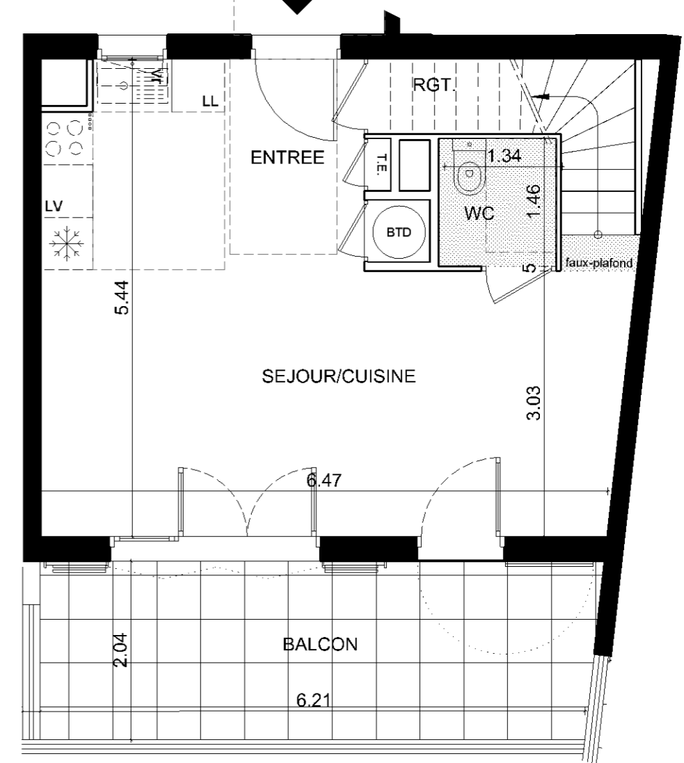
NIVEAU BAS
